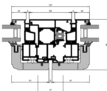
SEZIONE NODO CENTRALE
