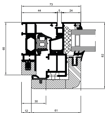
SEZIONE NODO LATERALE
