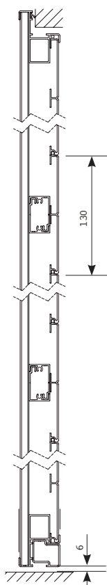
SEZIONE VERTICALE PORTA
