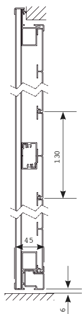
SEZIONE VERTICALE FINESTRA
